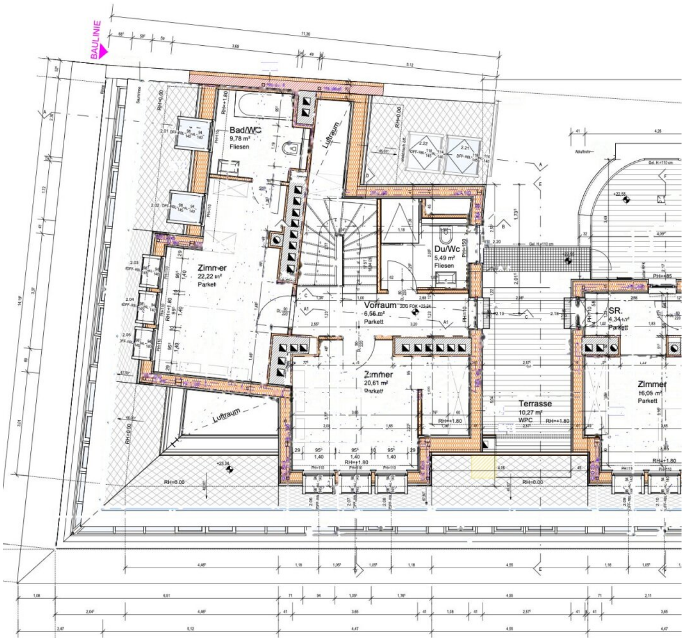
2. DACHGESCHOSS M 1 : 50
