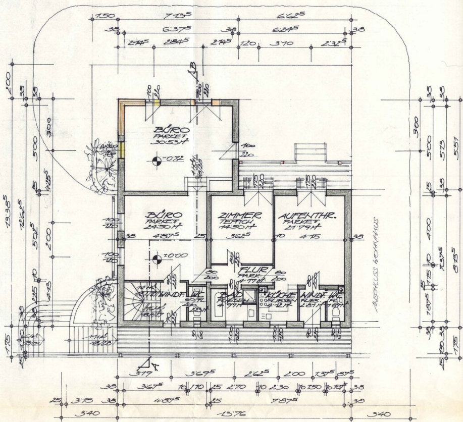
ERDGESCHOSS
