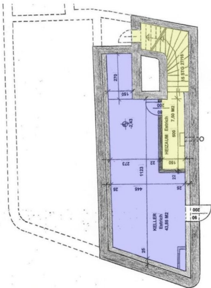
GRUNDRISS KELLER M 1:100
