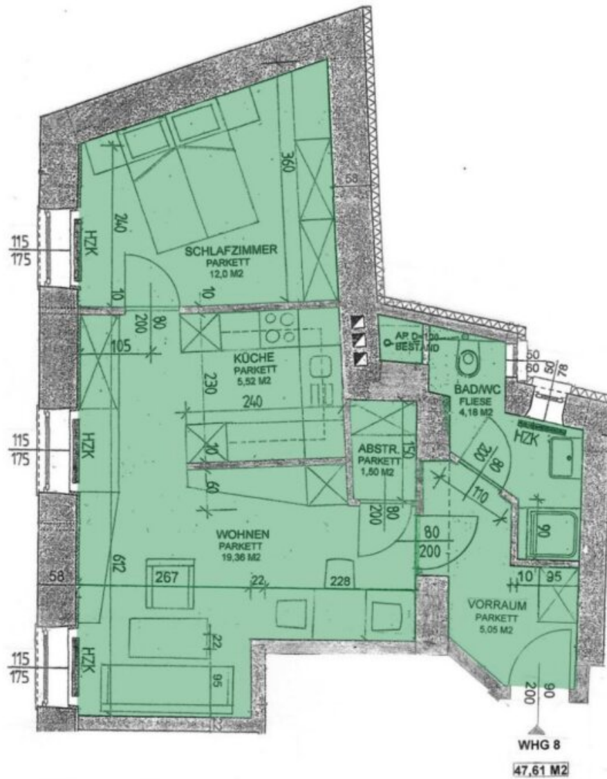
PARIFIZIERUNGSPLAN WHG 8 – 1.OG – M 1:50
