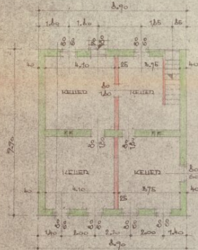
KELLERGESCHOSS
