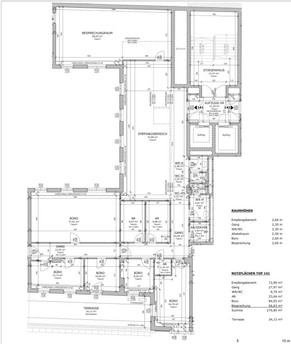
GRUNDRISS M 1:100 4. OBERGESCHOSS TOP 141
