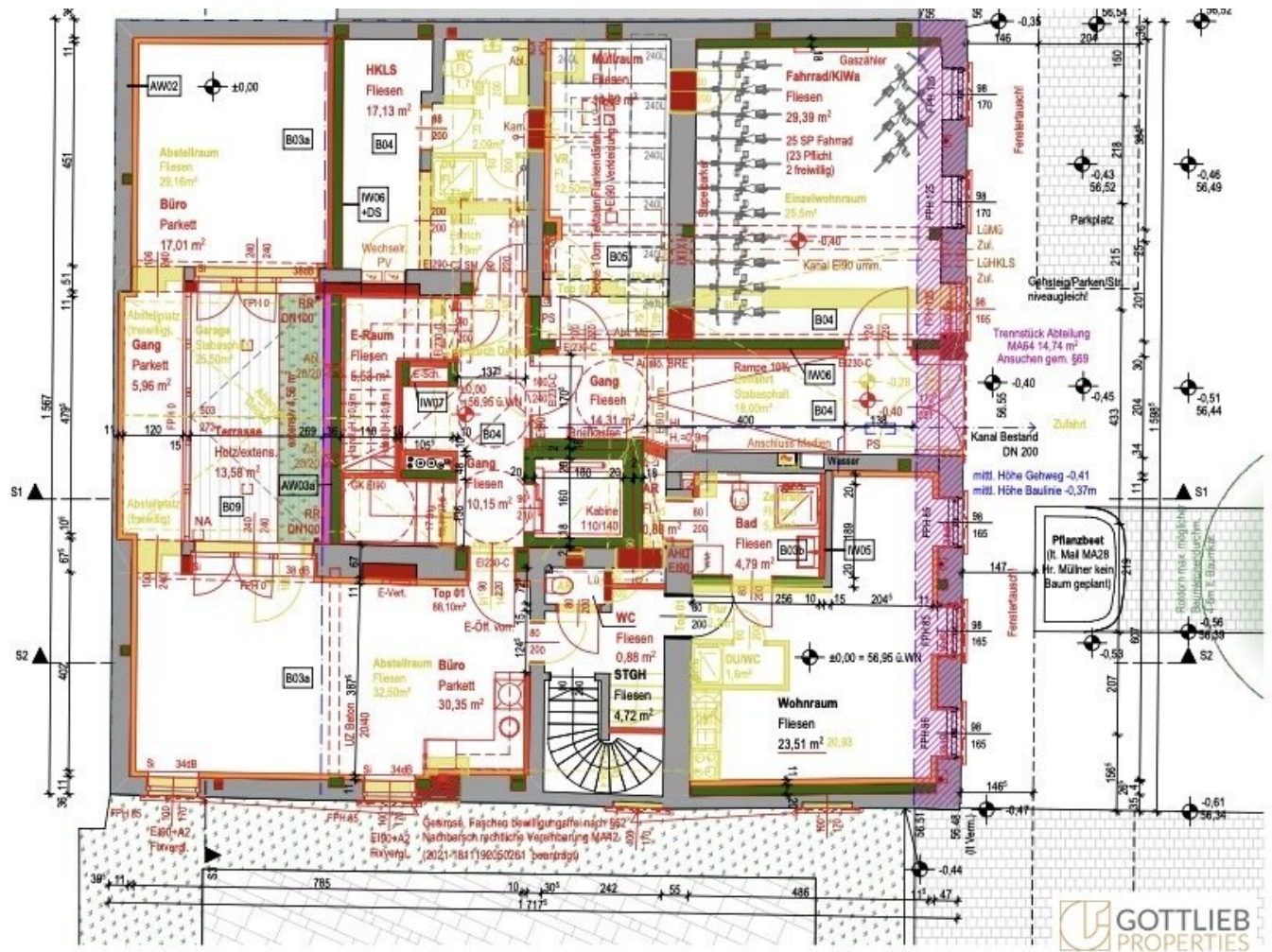
Erdgeschoss M.1.100
