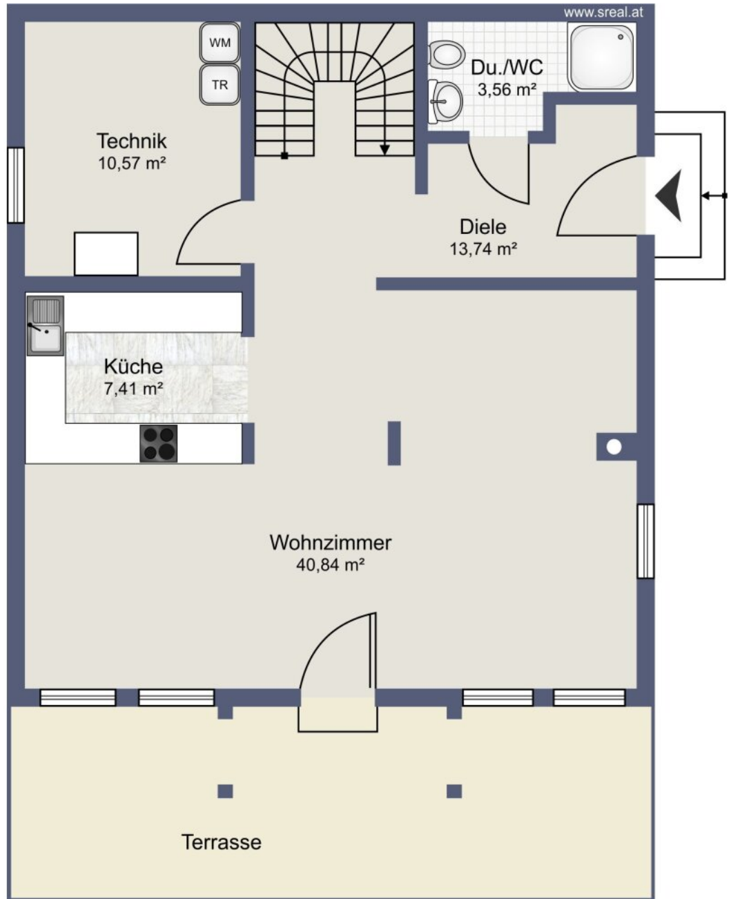
Skizze Erdgeschoss
