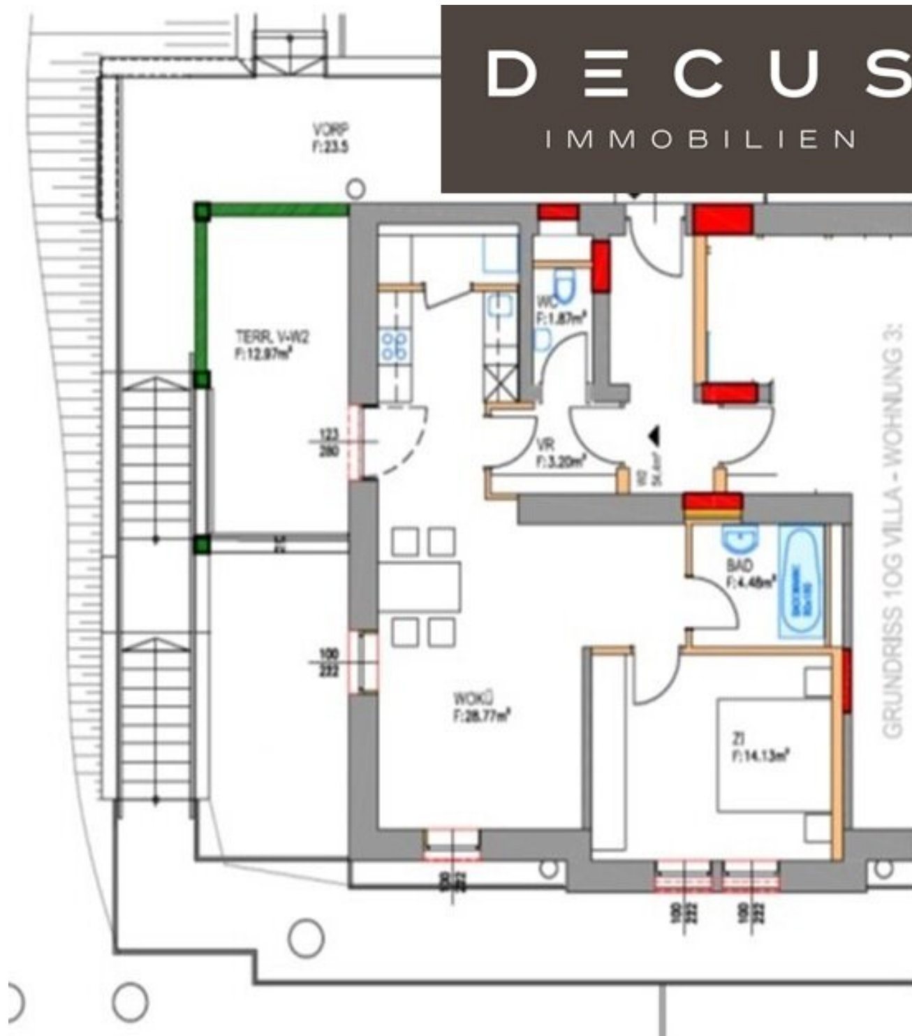
GRUNDRISS 1.OBERGESCHOSS :
