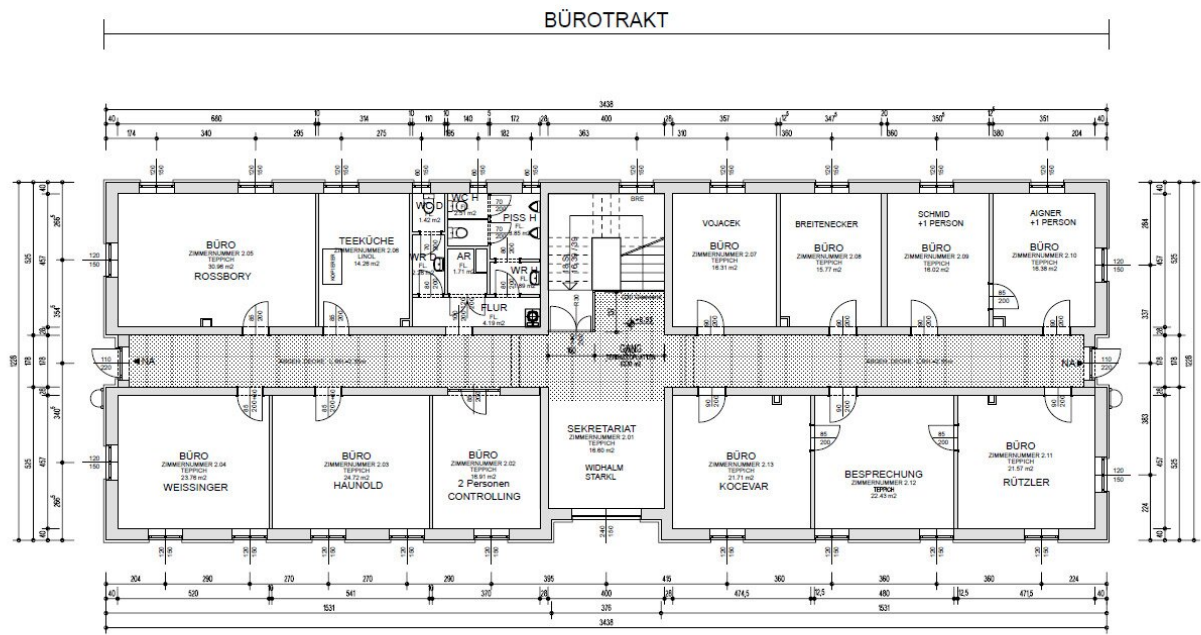
2. OBERGESCHOSS
