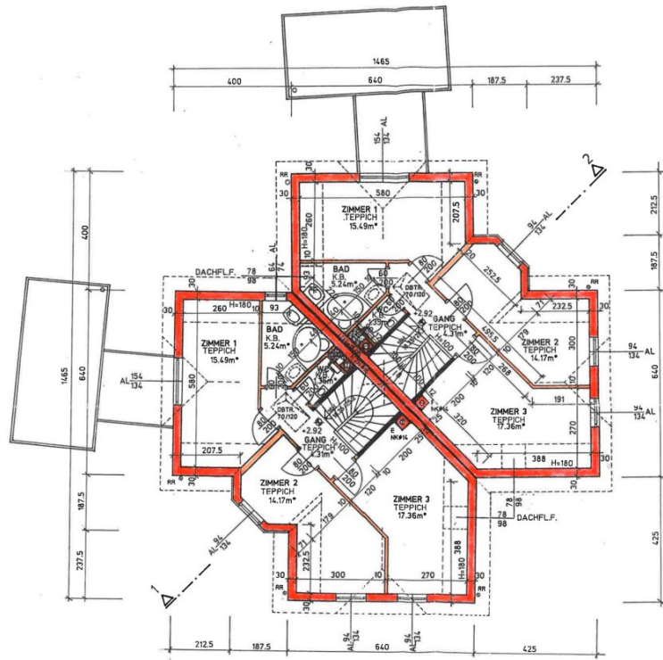
GRUNDRISS OBERGESCHOSS
