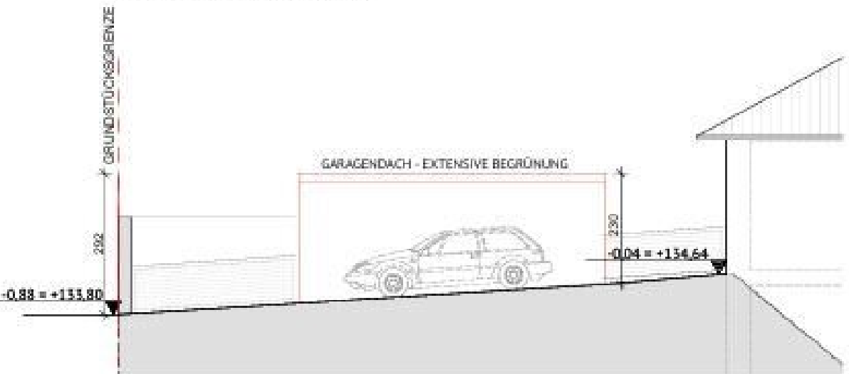
SÜD-WEST ANSICHT
