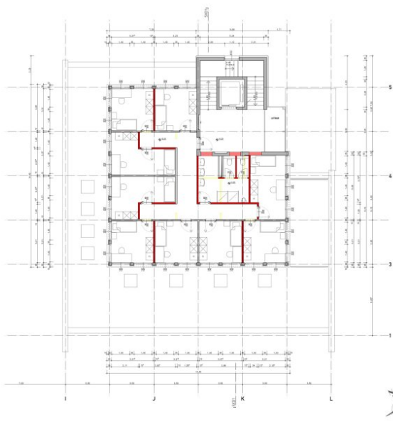
1. OBERGESCHOSS
