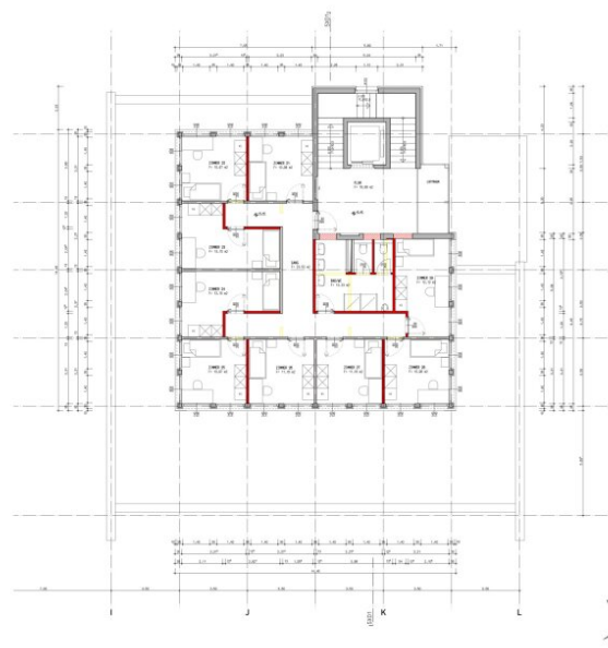
2. OBERGESCHOSS
