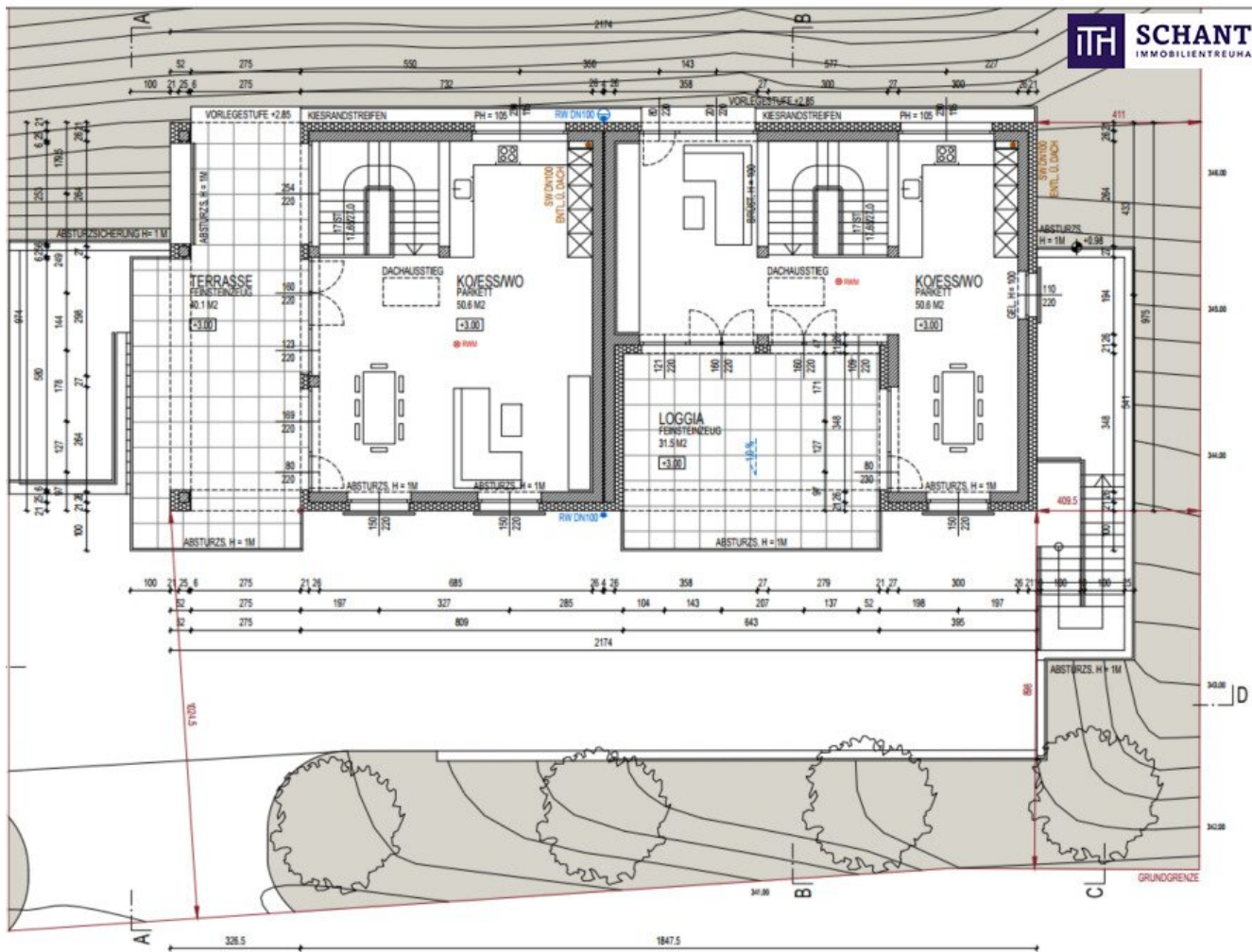
GRUNDRISS OBERGESCHOSS 1:100
