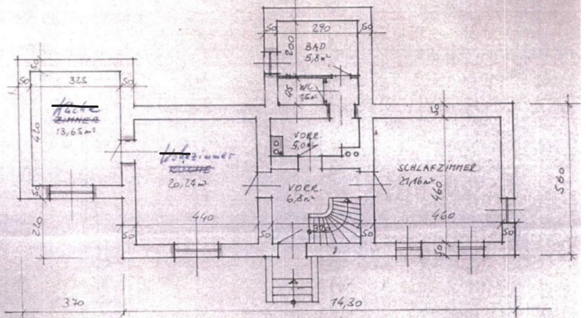
ERDGESCHOSS
