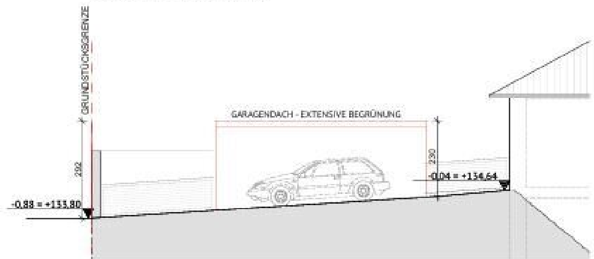
SÜD-WEST ANSICHT
