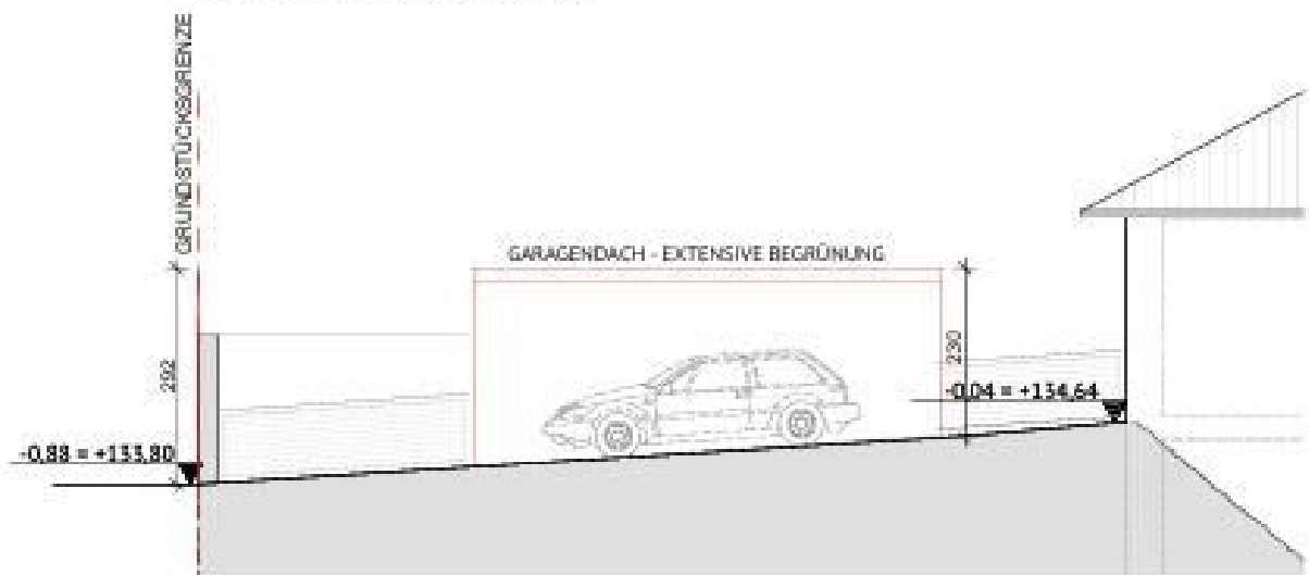
SÜD-WEST ANSICHT
