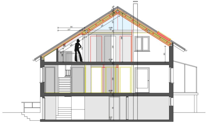
SCHNITT 2-2
