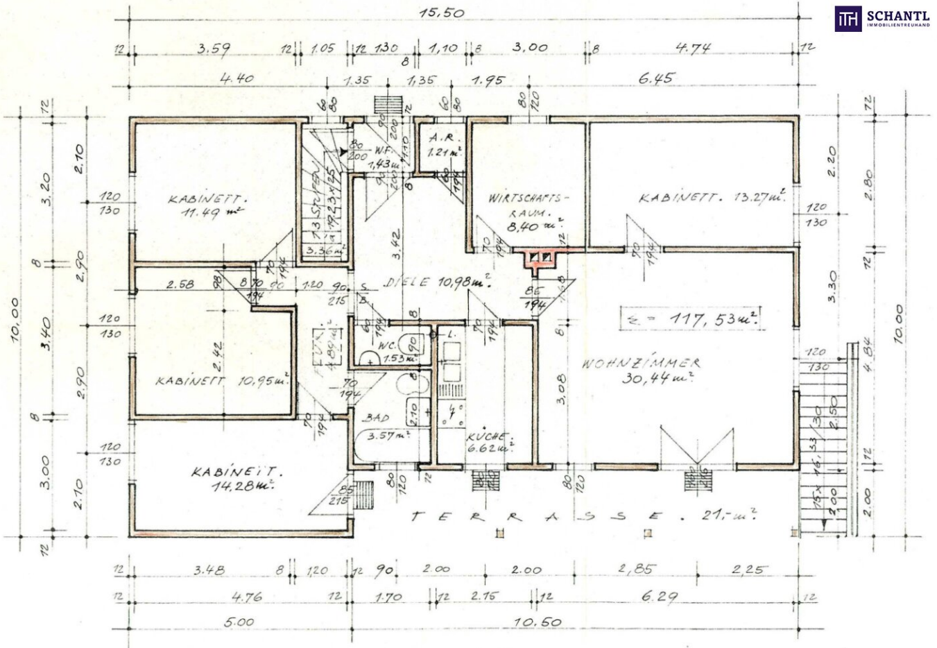
ERDGESCHOSS,
