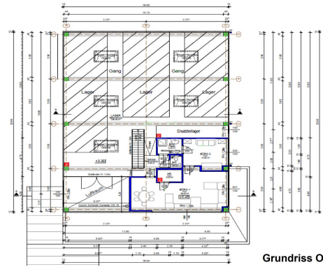
Grundriss OG
