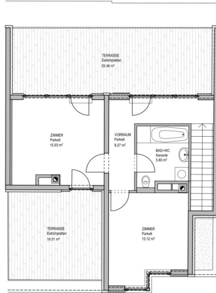
DACHGESCHOSS
