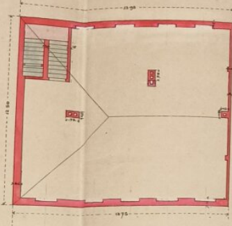
Dachboden
