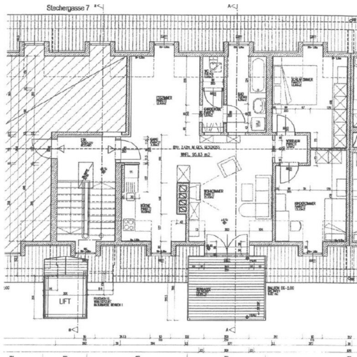
Grundriss DR Stechergasse 7 1:100
