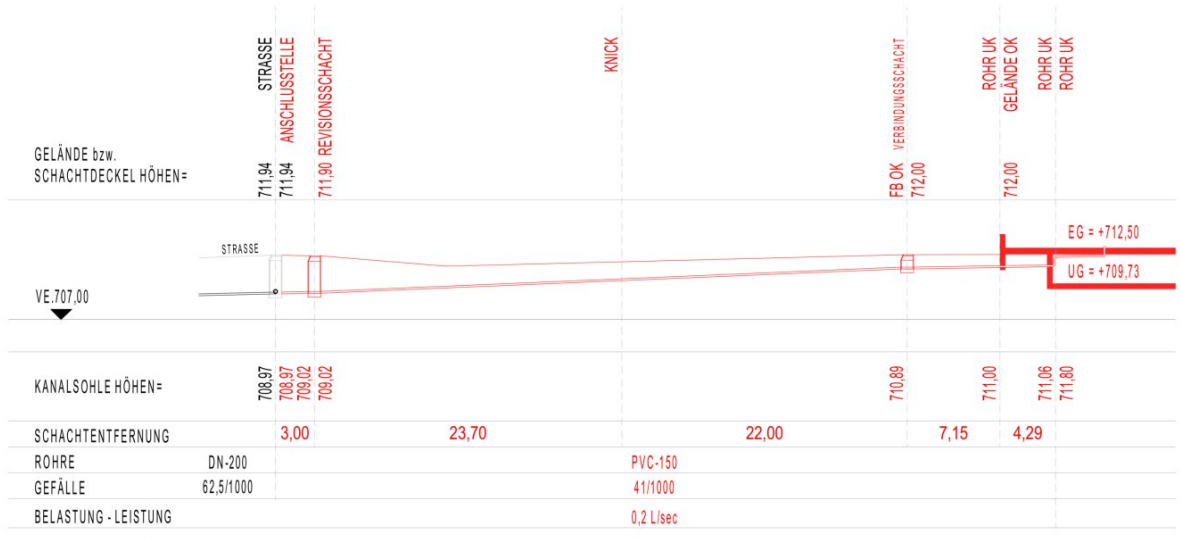
KANAL-HÖHENSCHNITT M 1:250
