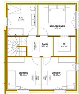
OBERGESCHOSS
