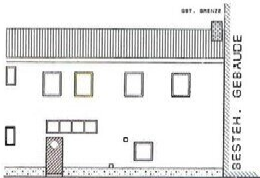
WESTANSICHT
