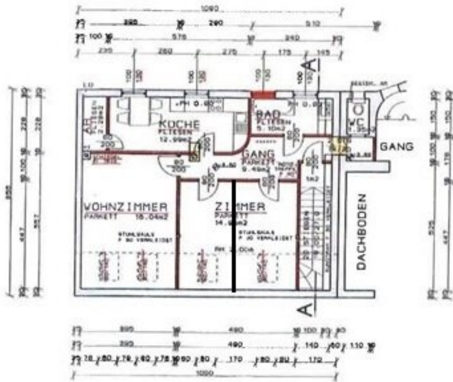
DACHGESCHOSS 63.20m 2
