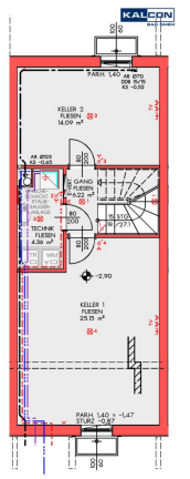
Kellergeschoss
