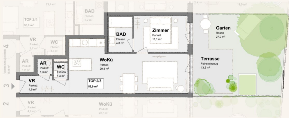
Grundriss Erdgeschoss
