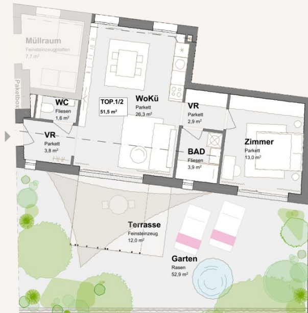
Grundriss Erdgeschoss
