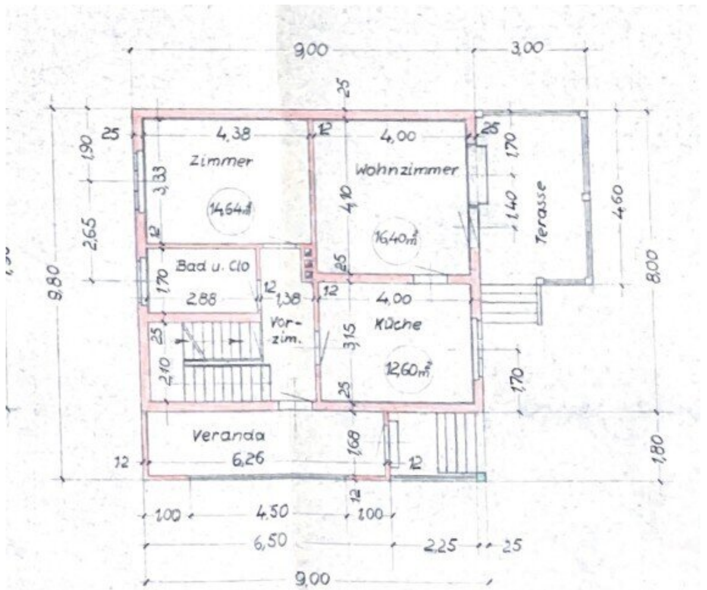
Erdgeschoss
