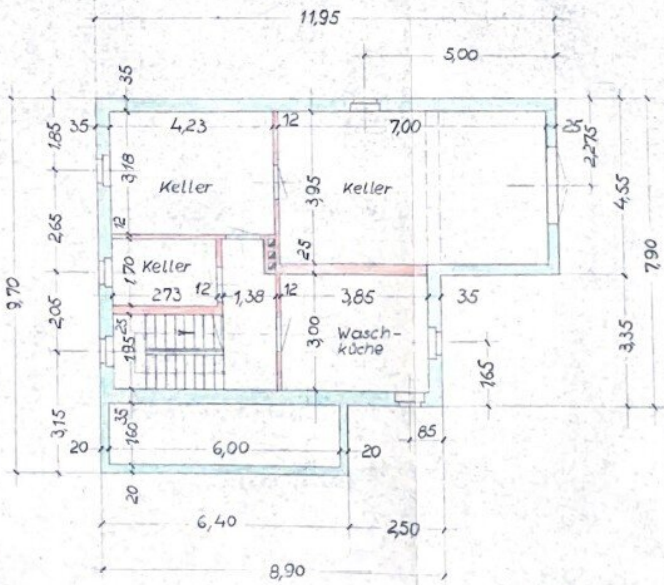
Kellergeschoß
