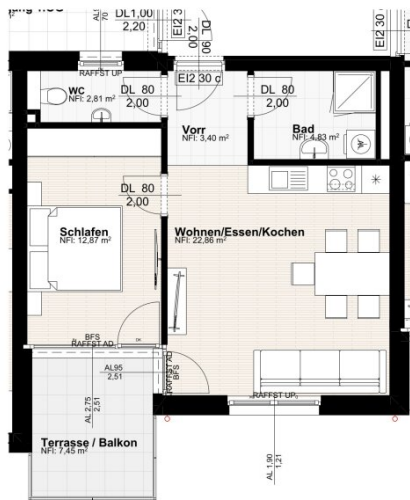
2. Obergeschoss
