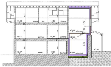
schnitt a-a
