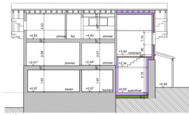
schnitt a-a
