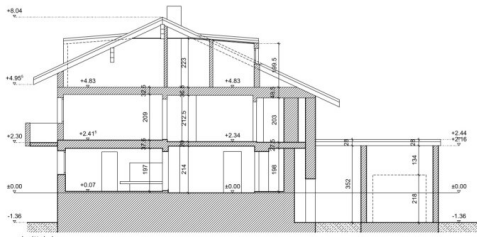
schnitt 1-1
