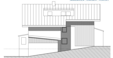
ostansicht
