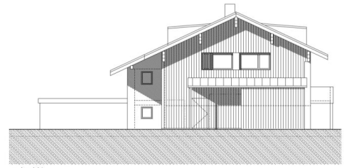
nordansicht
