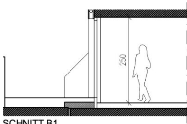
SCHNITT B1
