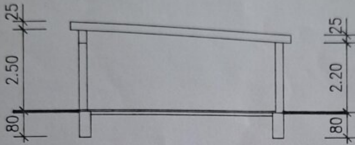
LANGSSCHNITT
