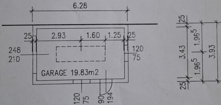
GRUNDRISS
