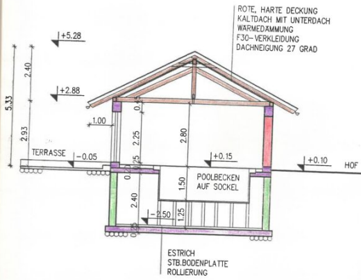
SCHNITT 3 - 3
