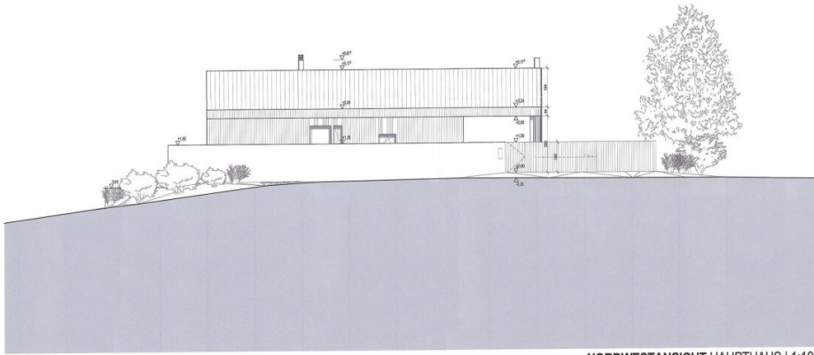
NORDWESTANSICHT HAUPTHAUS | 1:100
