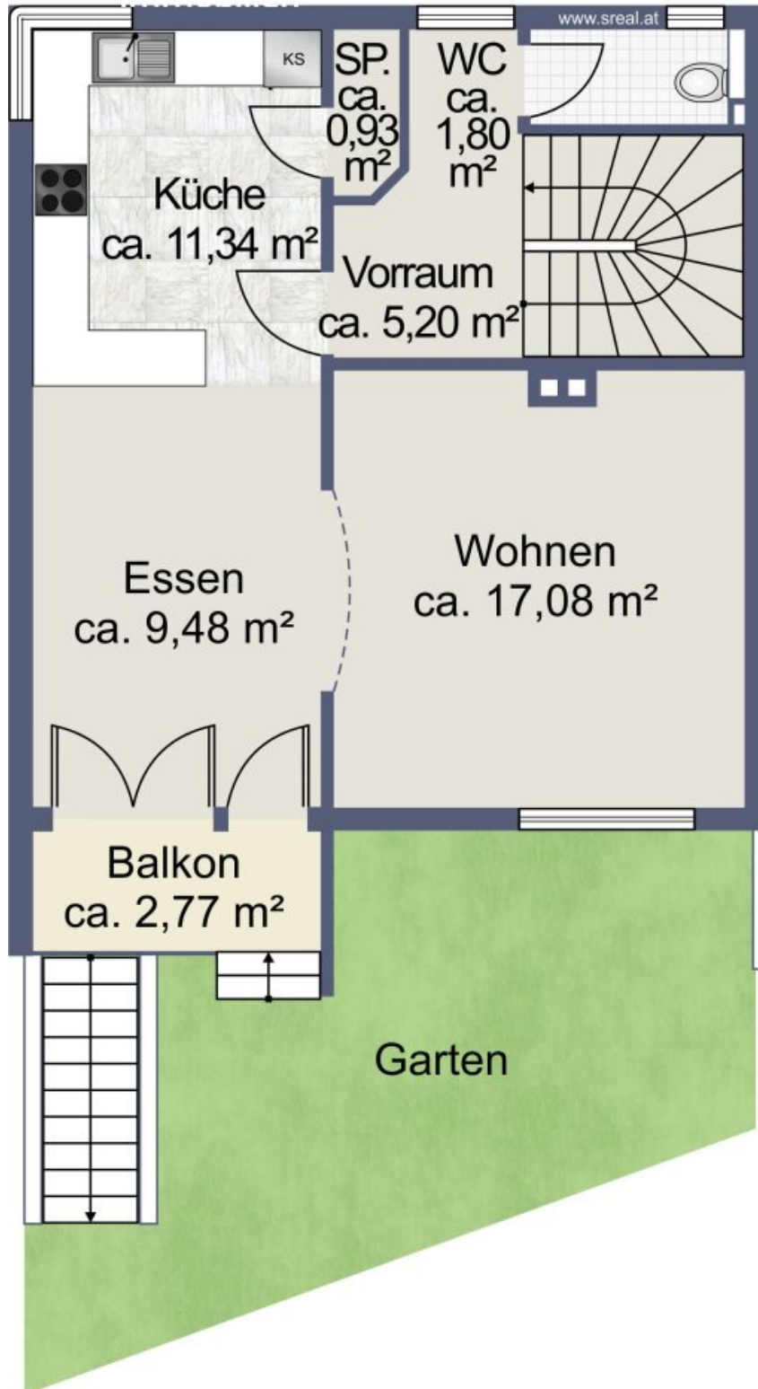
Skizze Erdgeschoss
