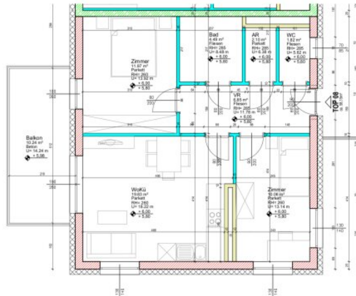
Planausschnitt 3.OBERGESCHOSS - Wohnung Planstand = Ausführungsplan M: 1:100
