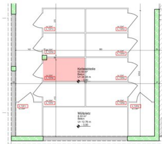
Planausschnitt KELLERGESCHOSS - Abteil TOP 08 - OST Planstand = Ausführungsplan M: 1:100
