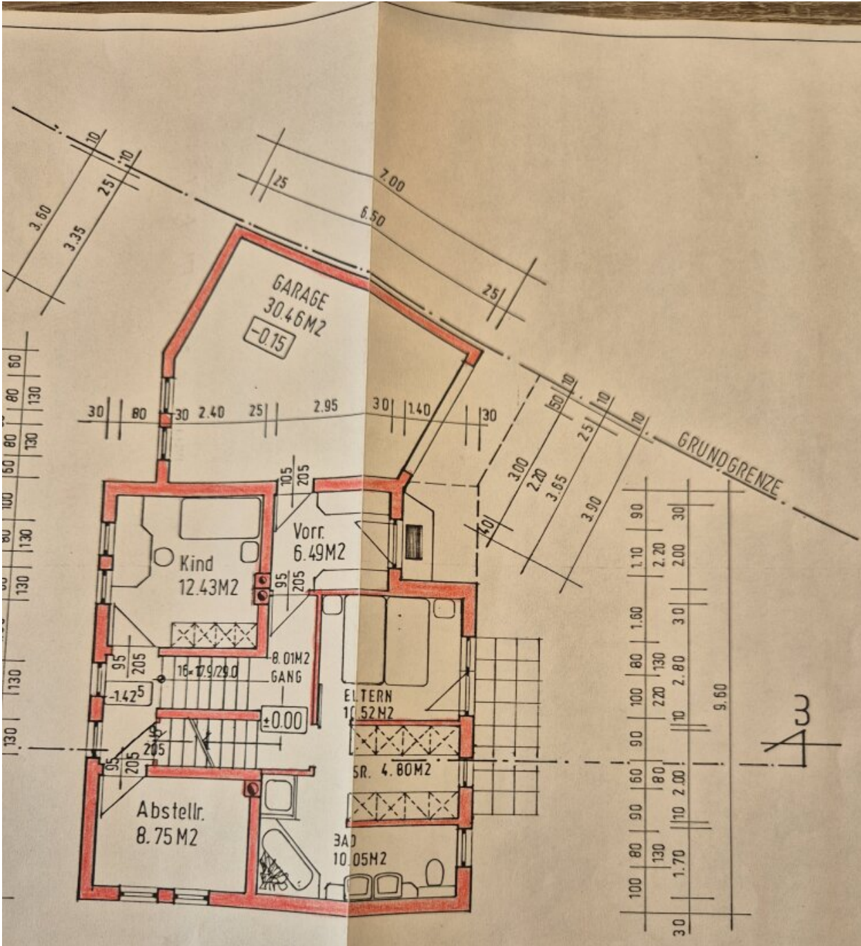
ERDGESCHOSS 1:100
