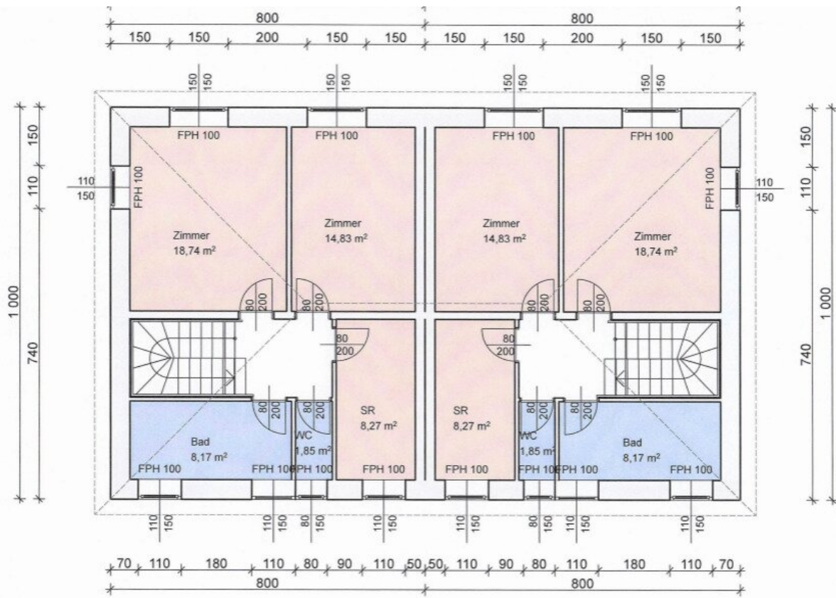
Obergeschoß Maßstab 1:100
