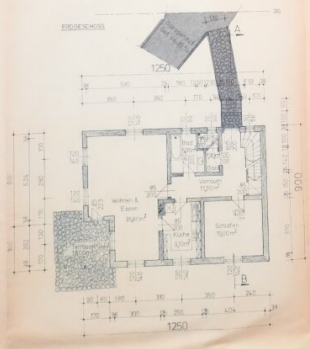
M. 1:100
