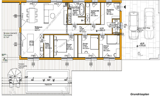
Grundrissplan
