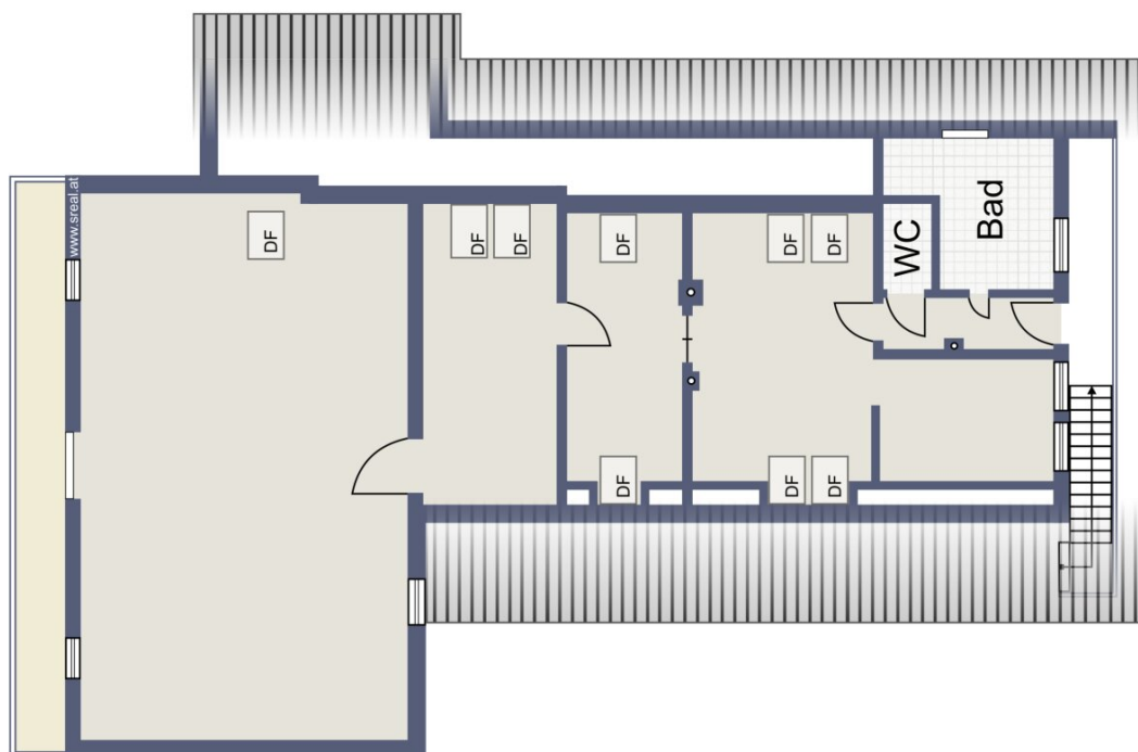
Skizze Obergeschoss
