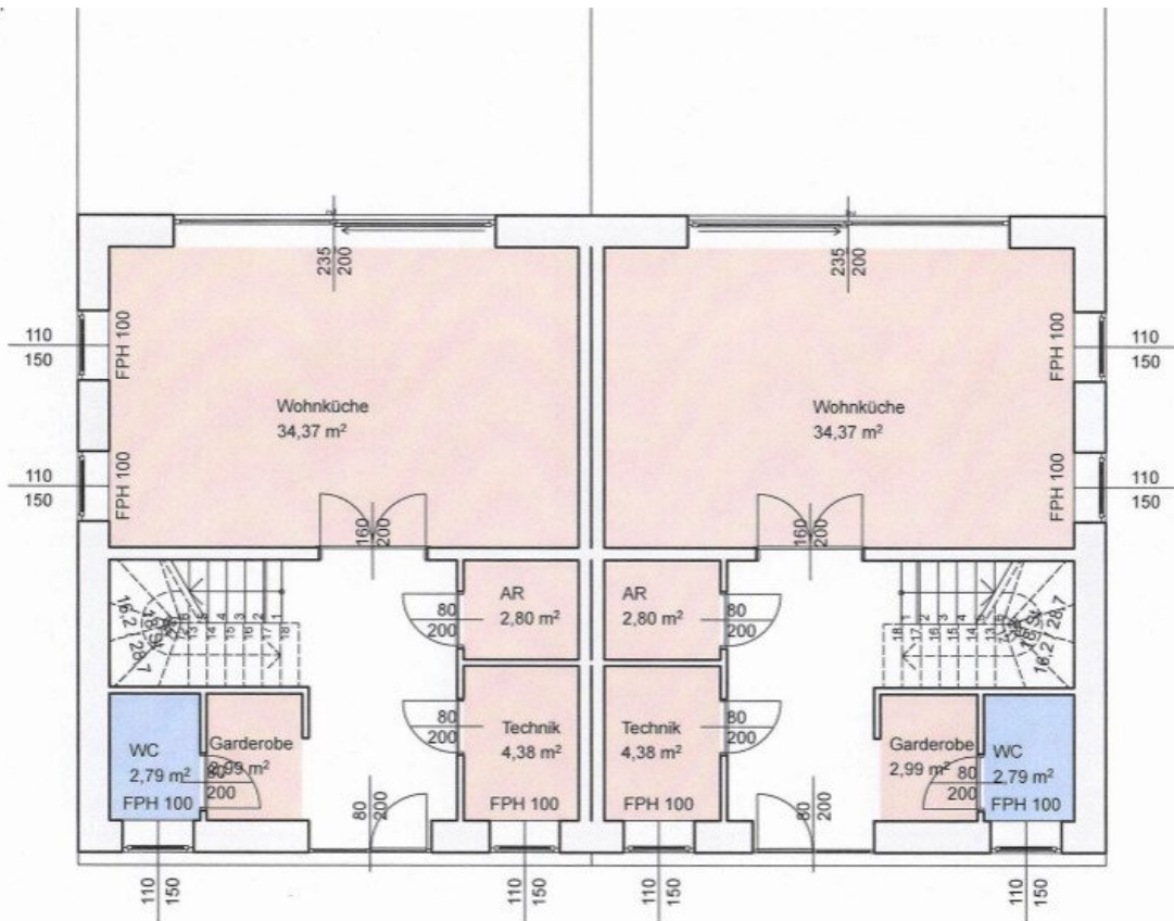
Erdgeschoß Maßstab 1:100
