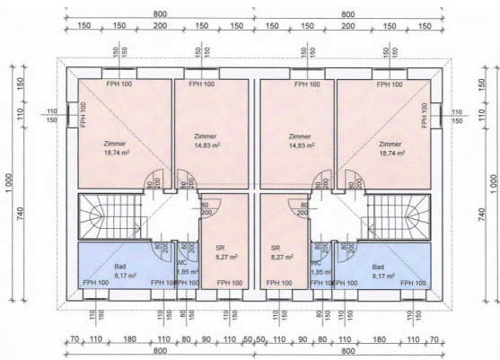
Obergeschoß Maßstab 1:100
