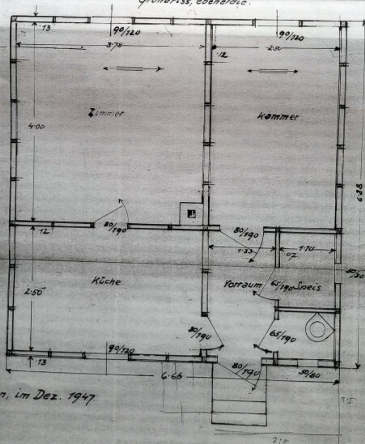
Grundriss, ebenerdig.
