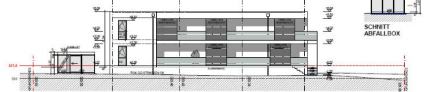
ANSICHT OST
