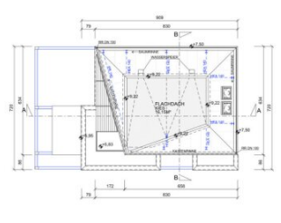
DACHDRAUFSICHT
