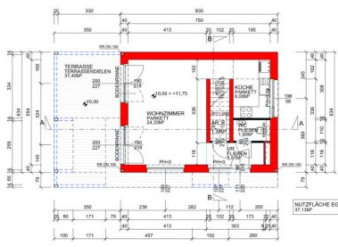
GRUNDRISS ERDGESCHOSS
