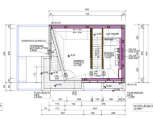
GRUNDRISS DACHGESCHOSS
