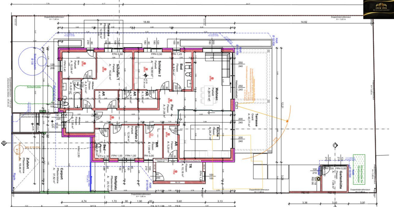
Grundriss EG
