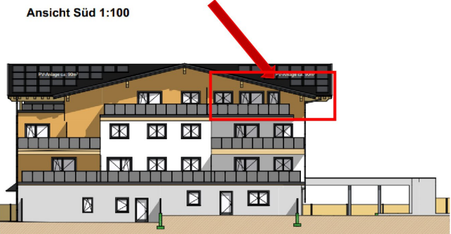
Ansicht Süd 1:100
