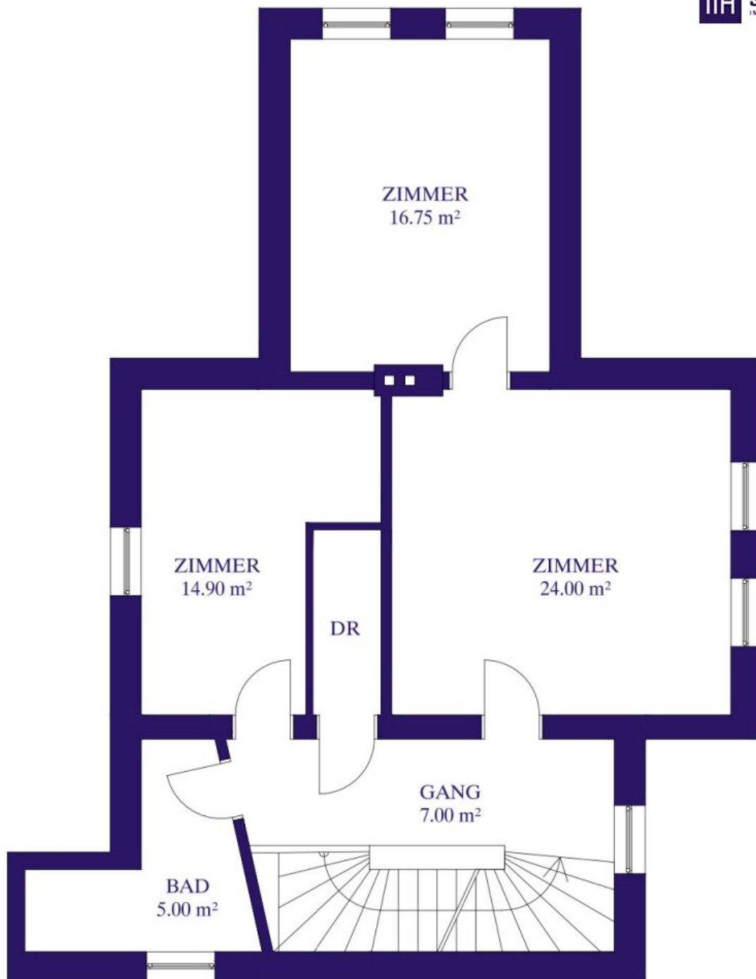
OBERGESCHOSS
