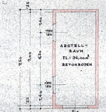
GRUNDRISZ
